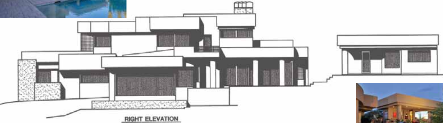
RIGHT ELEVATION
